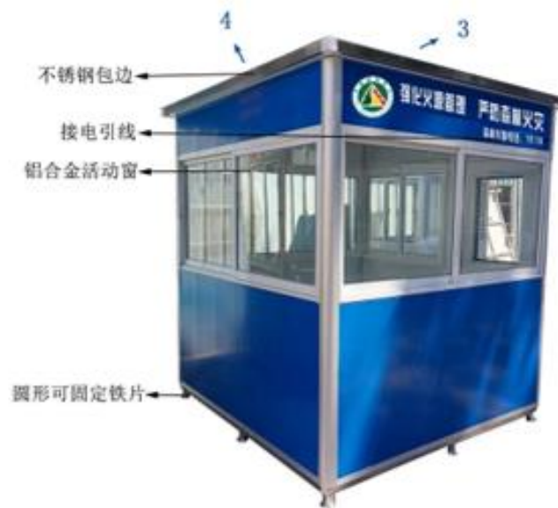
2.0*2.5*2.3保安亭外部配置图
